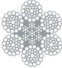
6X36WS + IWRC
