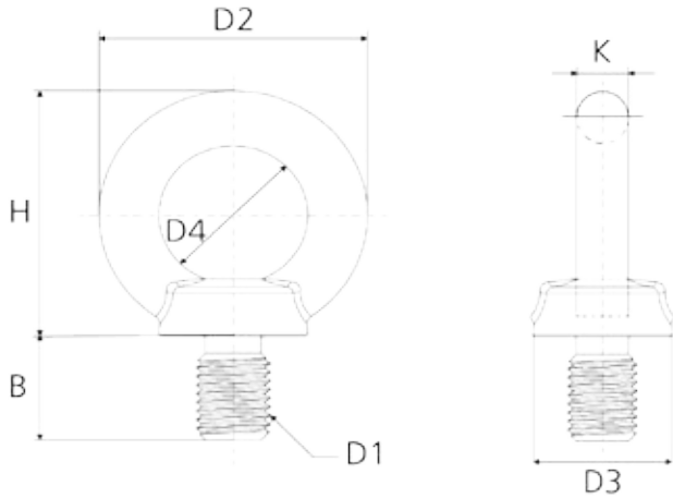
LIFTING EYE BOLT DIN 580:2010
