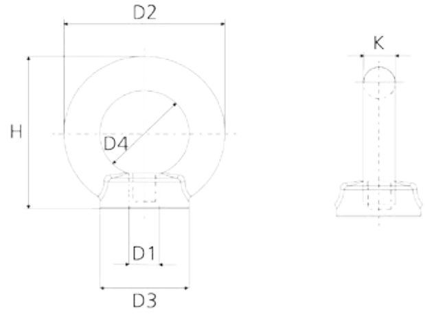
LIFTING EYE NUT DIN 582:2010
